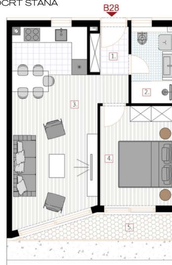
TLOCRT STANA
