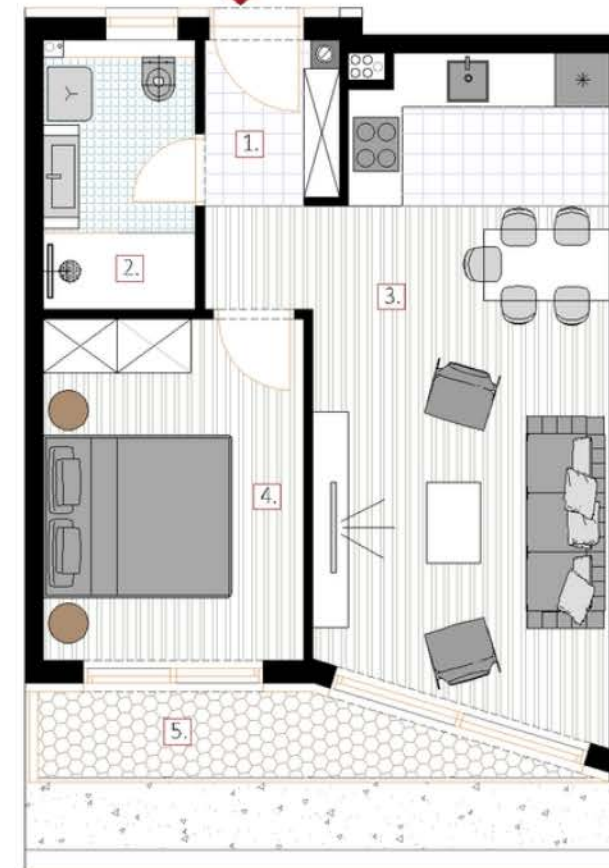
TLOCRT STANA B31
