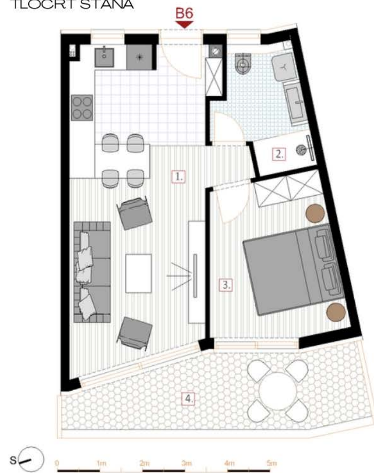
TLOCRT STANA
